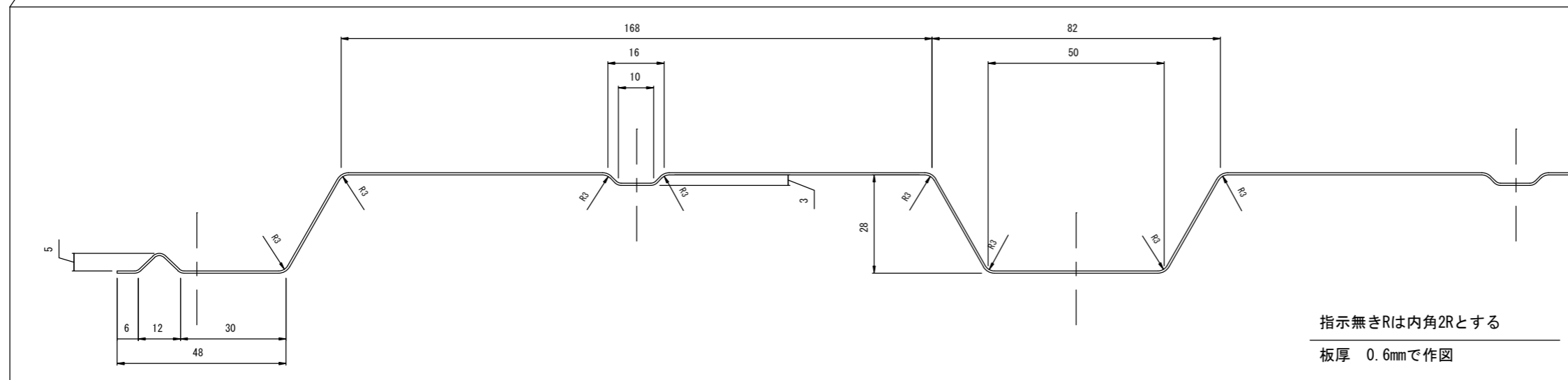
詳細図 1/1
